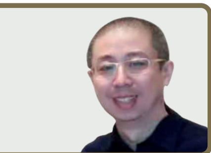
Biot WU
